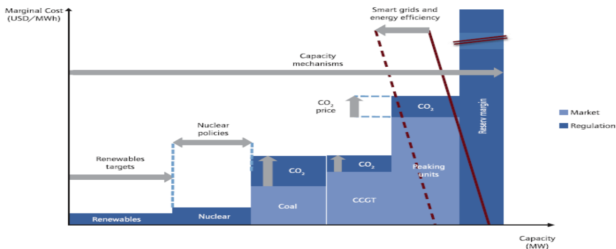
Διάγραμμα 1: Επίδραση πολιτικών στις εκπομπές CO 2
