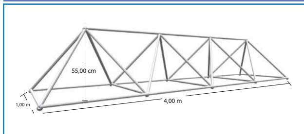
Χωροδικτύωμα
