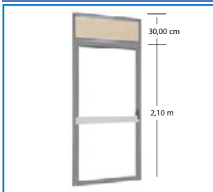
Πόρτα αλουμινίου
