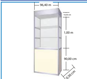
Βιτρίνα όψεως
